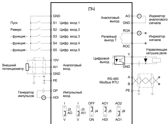
Рисунок 3 – Подключение управляющих клемм
