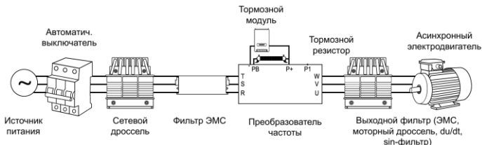
Рисунок 1 – Дополнительное оборудование
